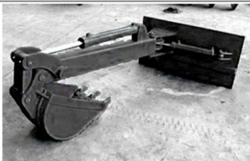
MINI SWIVEL DIGGER (MSD550)
